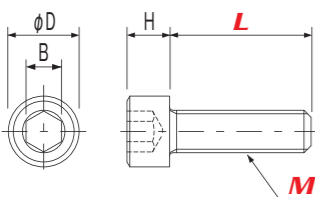
ポリカーボネート / 六角穴付ボルト Polycarbonate / Hexagon socket head cap bolt
